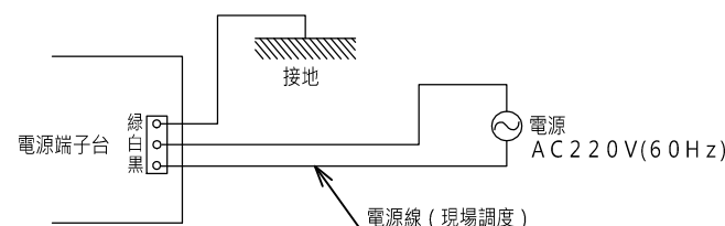
接線圖
