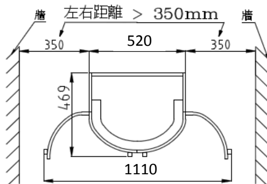
浴櫃寬度安裝尺寸示意圖
