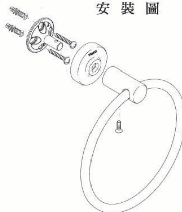
安裝圖
