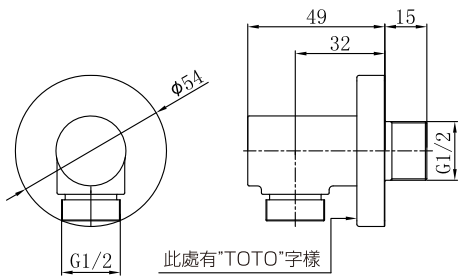
TBW01014B 蓮蓬頭出水口(圓形)
