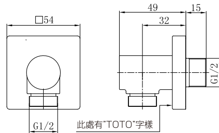
TBW02013B 蓮蓬頭出水口(方形)
