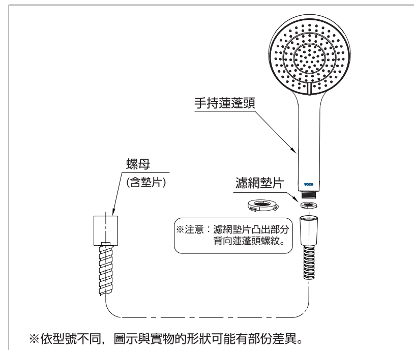
圖2：軟管的安裝
