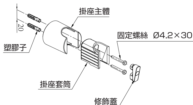
圖1：蓮蓬頭用掛座的安裝
