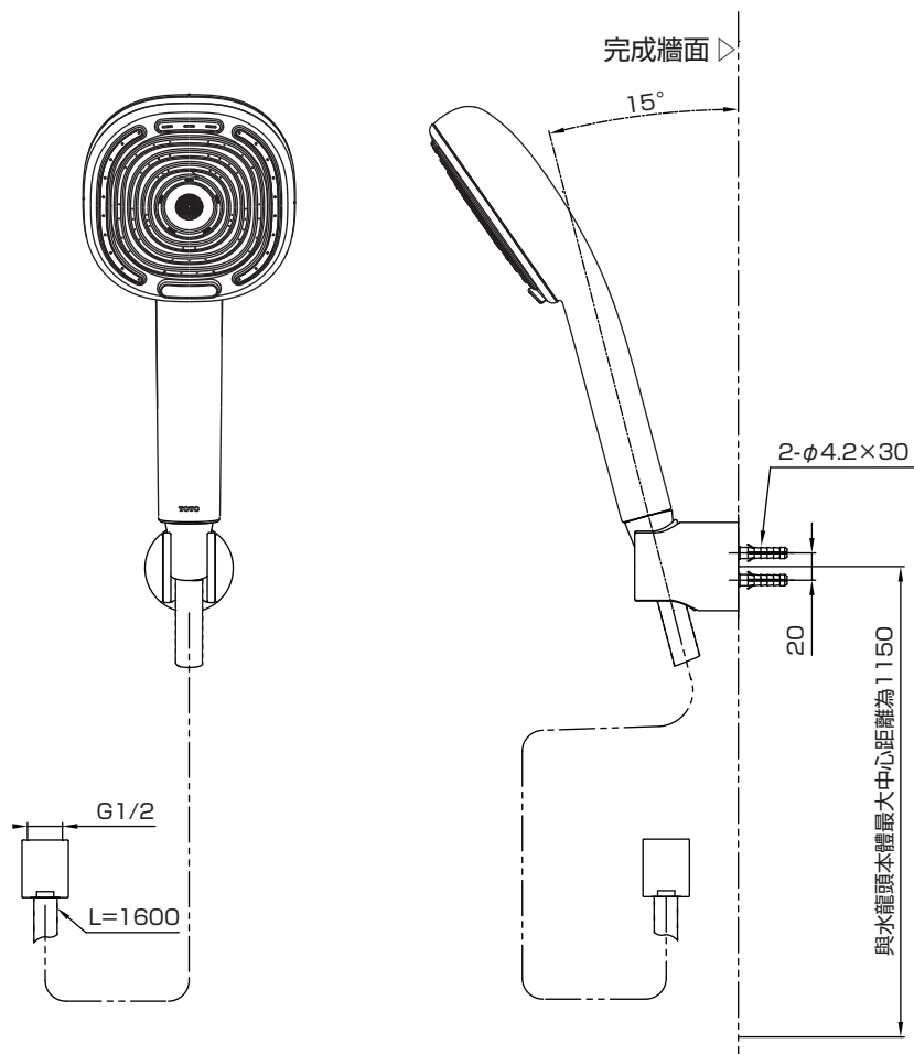
TBW15CEOP* 四段式手持蓮蓬頭
