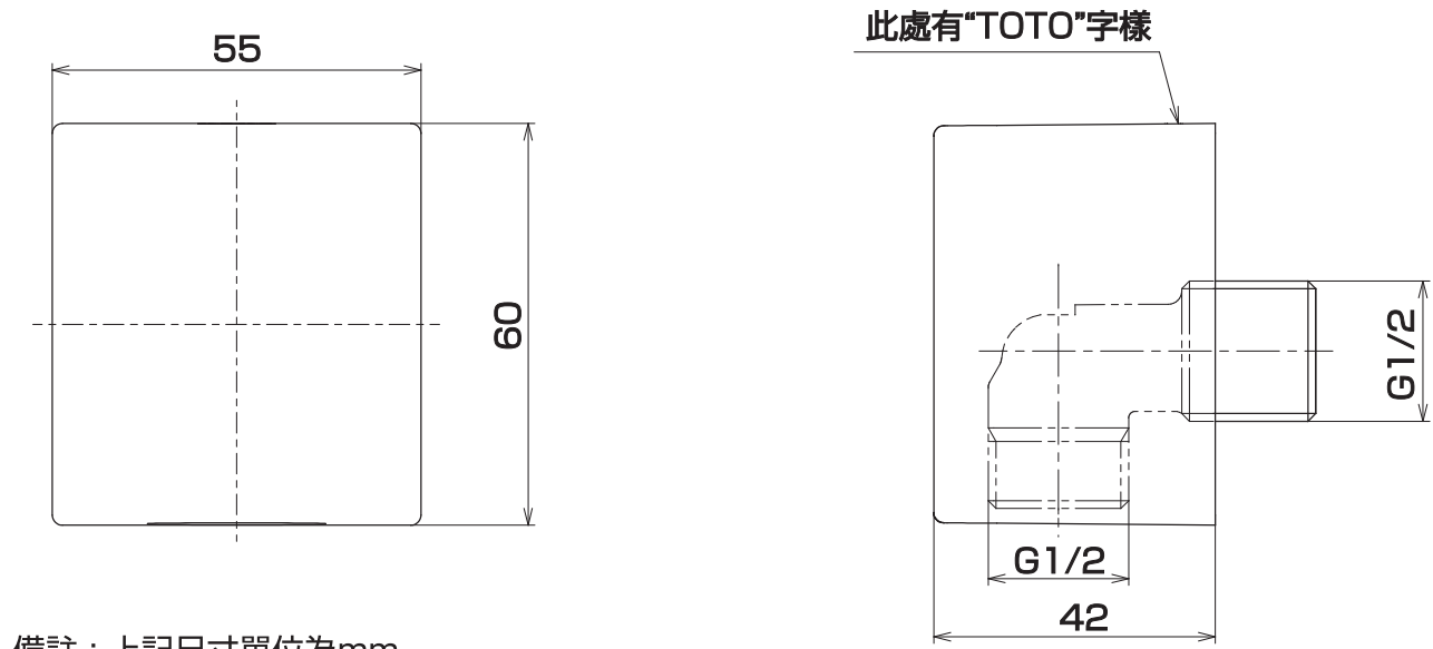
TBW160NO* 蓮蓬頭出水口
