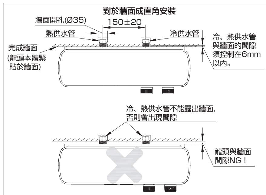
後彎腳的安裝示意圖
