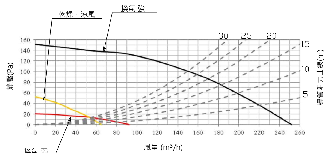
靜壓風量特性曲線
