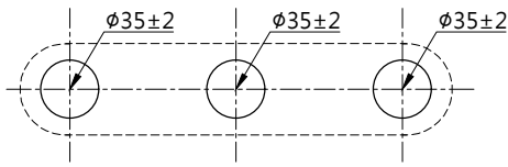
龍頭挖孔尺寸
