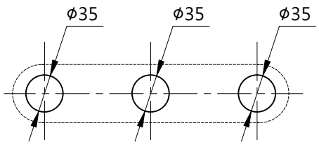
龍頭挖孔尺寸
