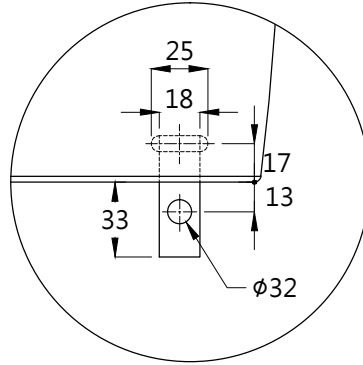
A部詳圖(1:3)
