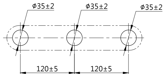
龍頭挖孔尺寸
