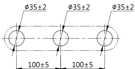
龍頭挖孔尺寸
