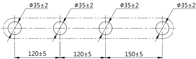
龍頭挖孔尺寸
