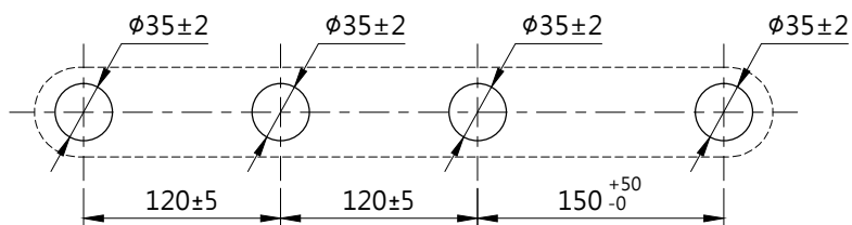
龍頭挖孔尺寸
