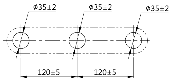
龍頭挖孔尺寸
