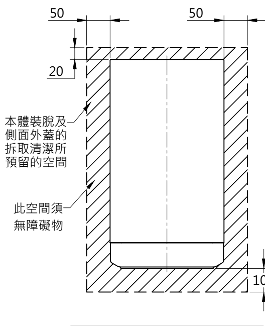
壁面直接安裝
