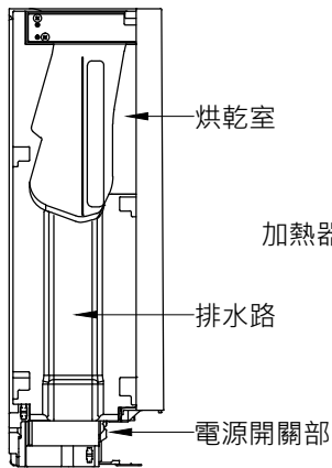
拆下側面外蓋和盛水盤
