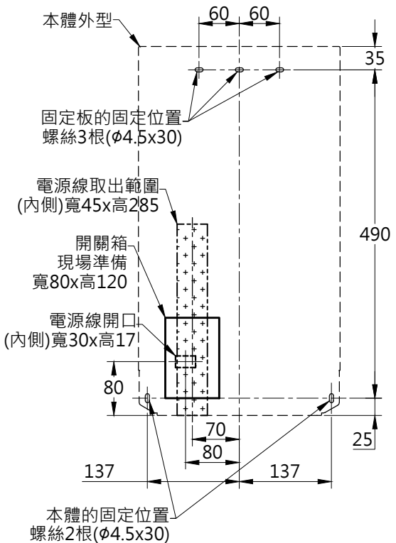
安裝用固定板
