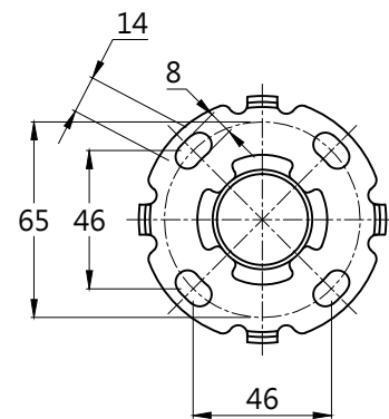
安裝底座放大圖(5:1)
