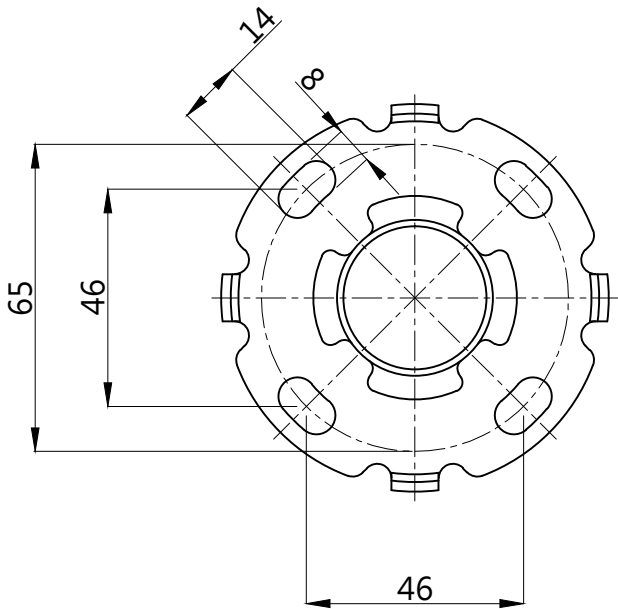
安裝底座放大圖( 5:1 )
