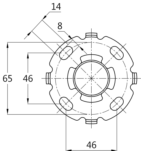
安裝底座放大圖( 5:1 )
