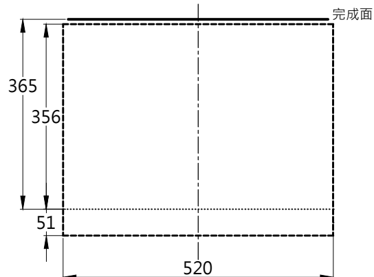
LW1316CBTW 檯面裁切尺寸
