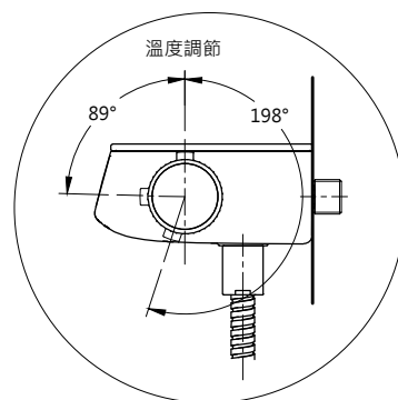
局部視圖B (圖面比例 2:1)
