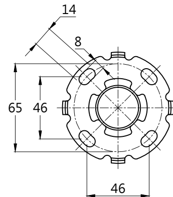
安裝底座放大圖(5:1)
