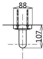
安裝底座細部(1:2)
