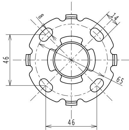
安裝底座細部(1:2)
